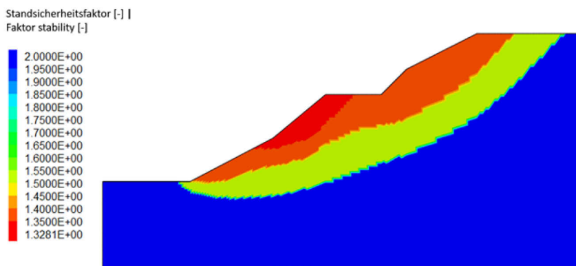
Abbildung 4-1: Standsicherheitsfaktor einer generischen Böschung (Itasca Consulting Group inc., 2019).
