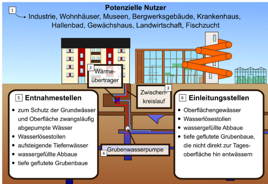
Abbildung 6-1: Schematische Darstellung des grundlegenden Prinzips zur energetischen Grubenwassernutzung sowie mögliche Entnahme-, Einleitungsstellen und potenzielle Nutzer (nach Oppelt 2020a).
